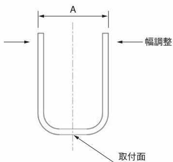
図 1 U 曲げ図面
