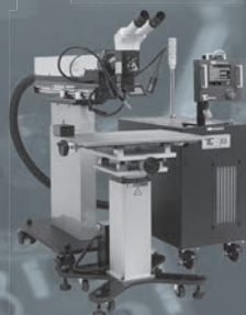
Laser Welder TL Series TL-50/150/200 TL シリーズ
