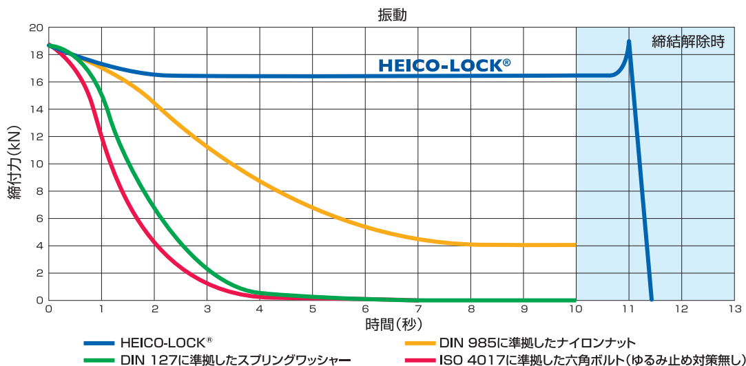
グラフ：振動テスト DIN65151 / DIN25201-4で実証された軸力損失プロセス
