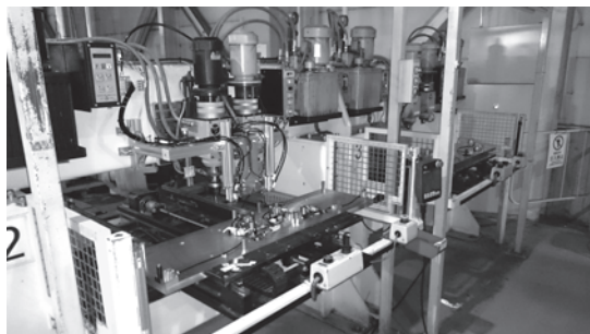
写真2 LBP シャーシ自動加工ラインの自動かしめ装置
