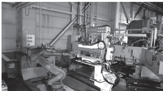
写真1 LBP シャーシ自動加工ライン
