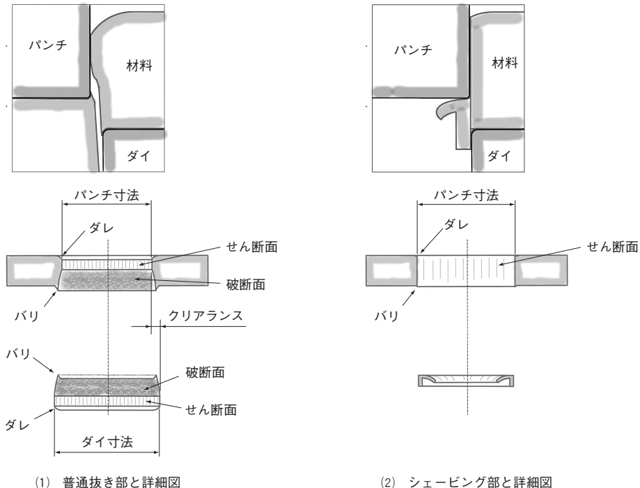
図1 普通抜きとシェービングの概要図
