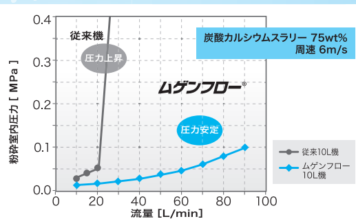
■ 粉碎室内の圧力変化
