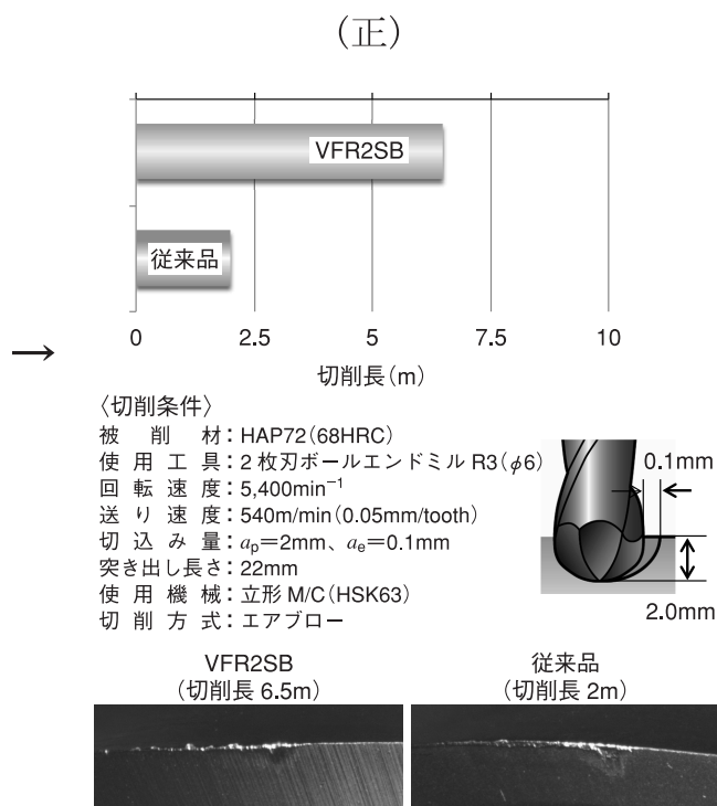
図7 HAP 72 (68 HRC) の工具寿命比較
