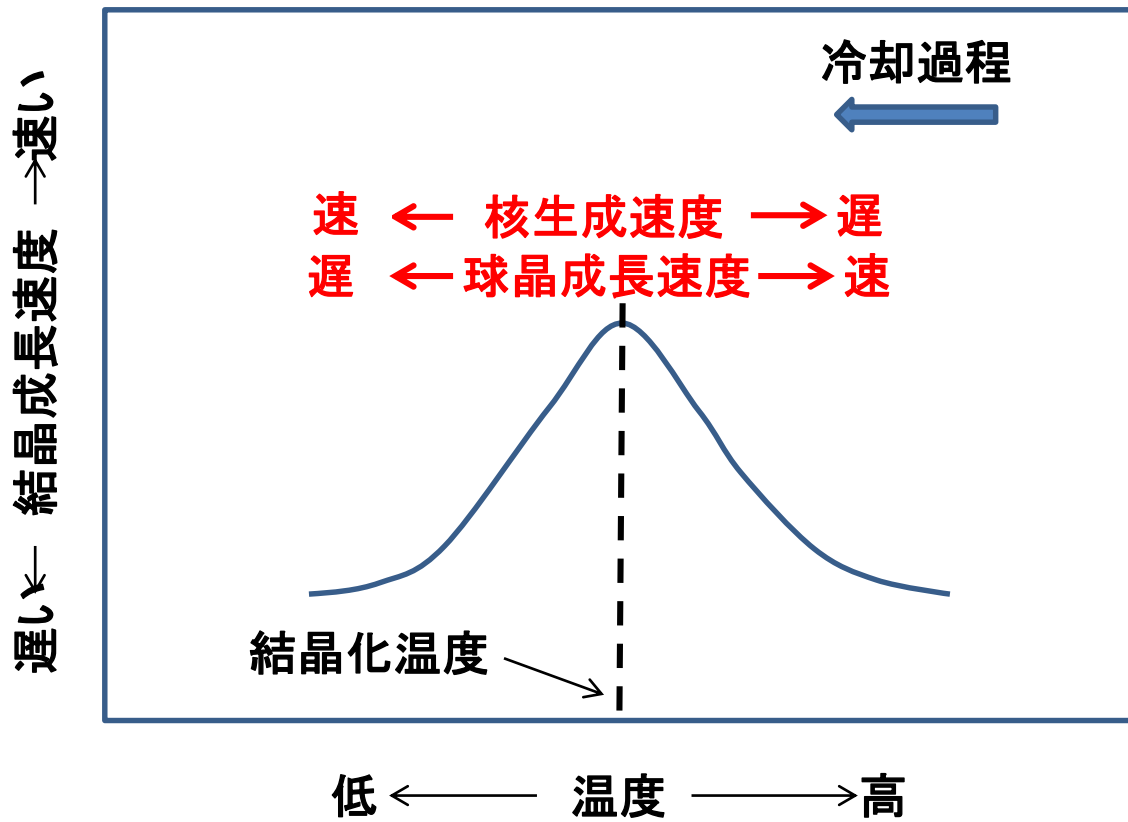
図1. 17 結晶成長速度の概念図
