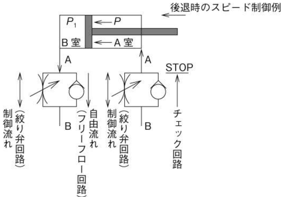
図3-47 速度制御の原理 (メータイン回路)
